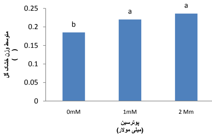
شکل ۲. تأثیر پوترسین بر وزن خشک گل همیشه‌بهار
