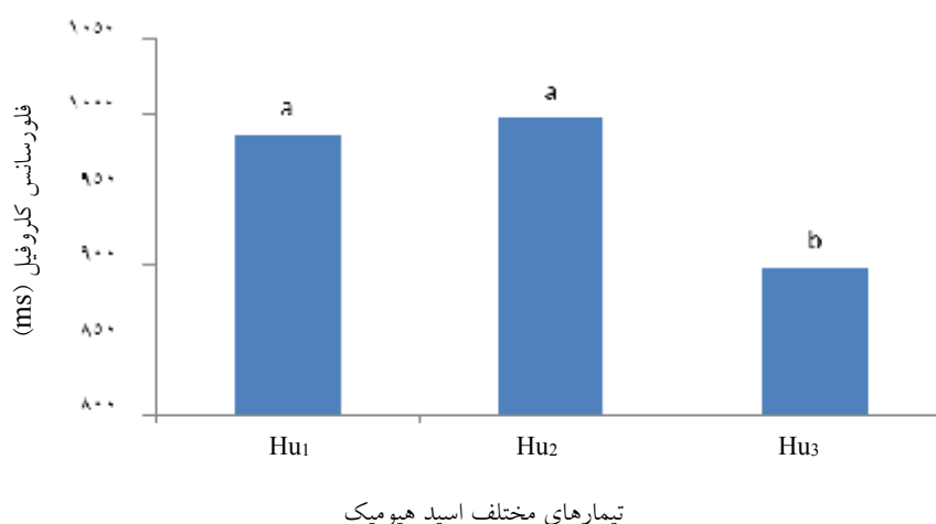
شکل ۷. مقایسه میانگین تأثیر غلظت‌های مختلف اسید هیومیک بر میزان فلورسانس حداکثر
