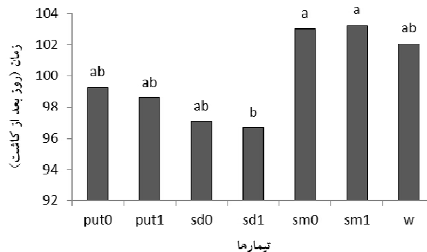
شکل ۱. مقایسه میانگین اثر تیمارهای پلی آمینی بر زمان گل دهی (میانگین تعداد روز از زمان کاشت تا ظهور ساقه گل دهنده) در فریزا. تیمارها شامل: پوترسین ۰/۵ میلی مولار (put0)، پوترسین ۱ میلی مولار (put1)، اسپرمیدین ۰/۵ میلی مولار (sd0)، اسپرمیدین ۱ میلی مولار (sd1)، اسپرمین ۰/۵ میلی مولار (sm0)، اسپرمین ۱ میلی مولار (sm1) و آب مقطر (w) هستند. در این شکل، ستون های دارای حداقل یک حرف مشترک، اختلاف معنی داری از نظر آماری با یکدیگر ندارند.
